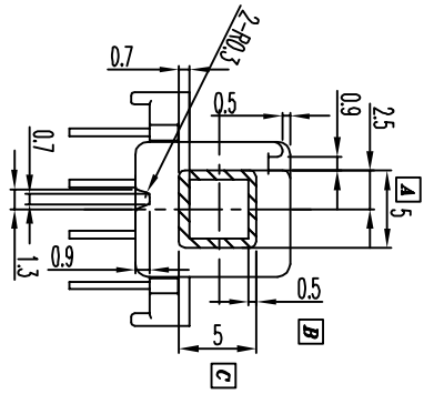
SEC A-A
